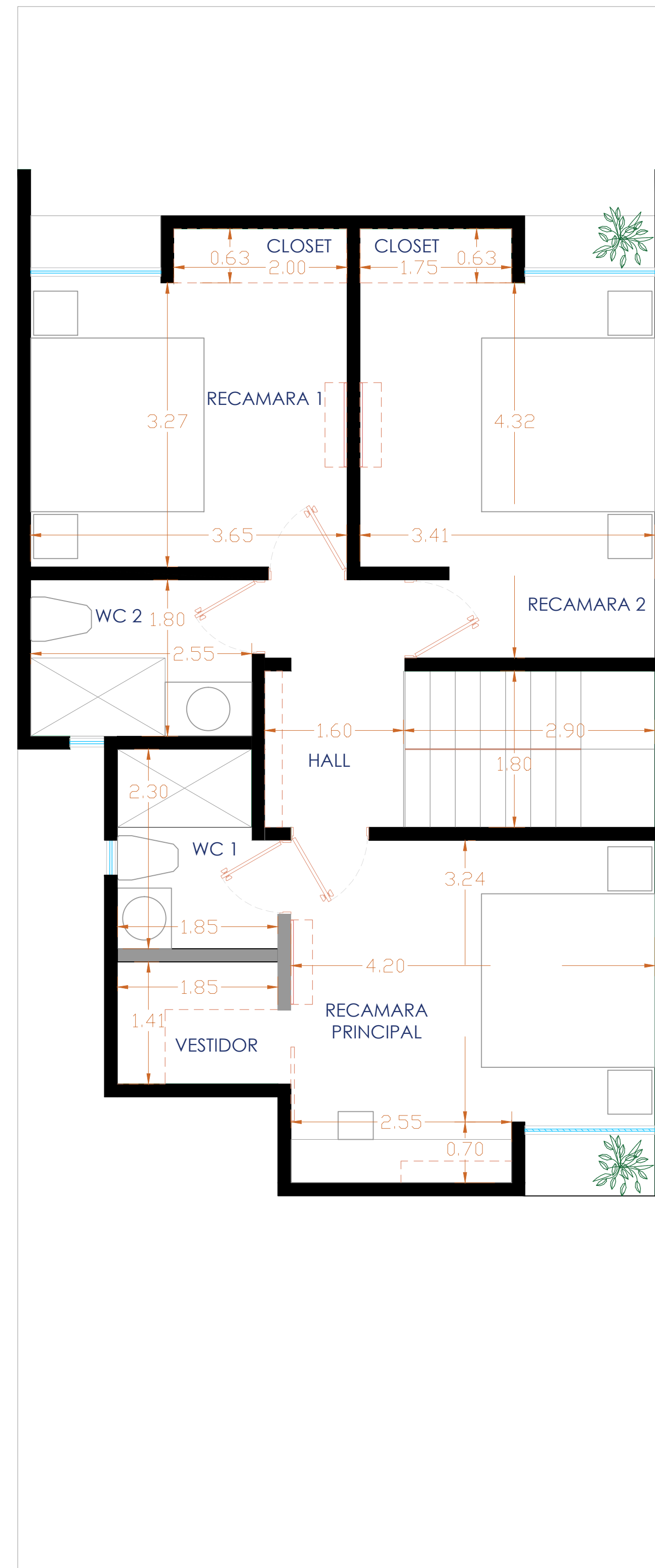
Primer nivel
