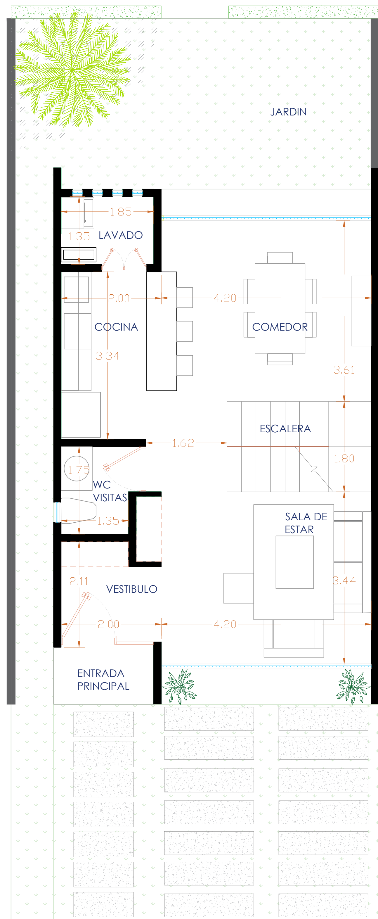
Planta baja
